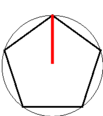
Mnohoúhelník vepsaný
