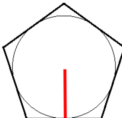
Mnohoúhelník opsaný
